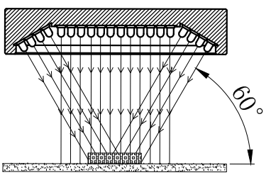
照明示意图
