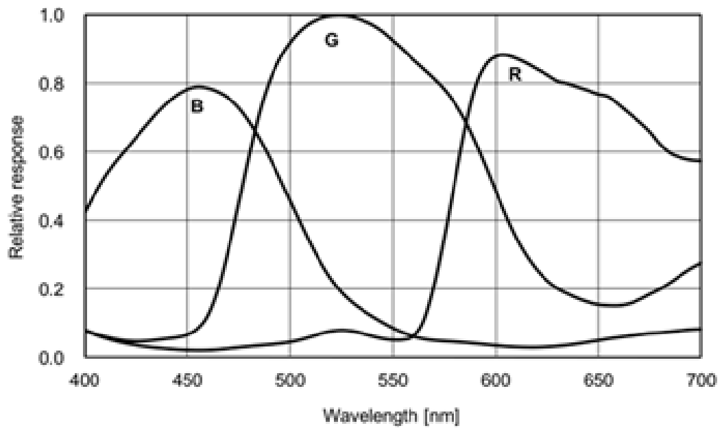
MER2-1220-32U3C 光谱曲线
