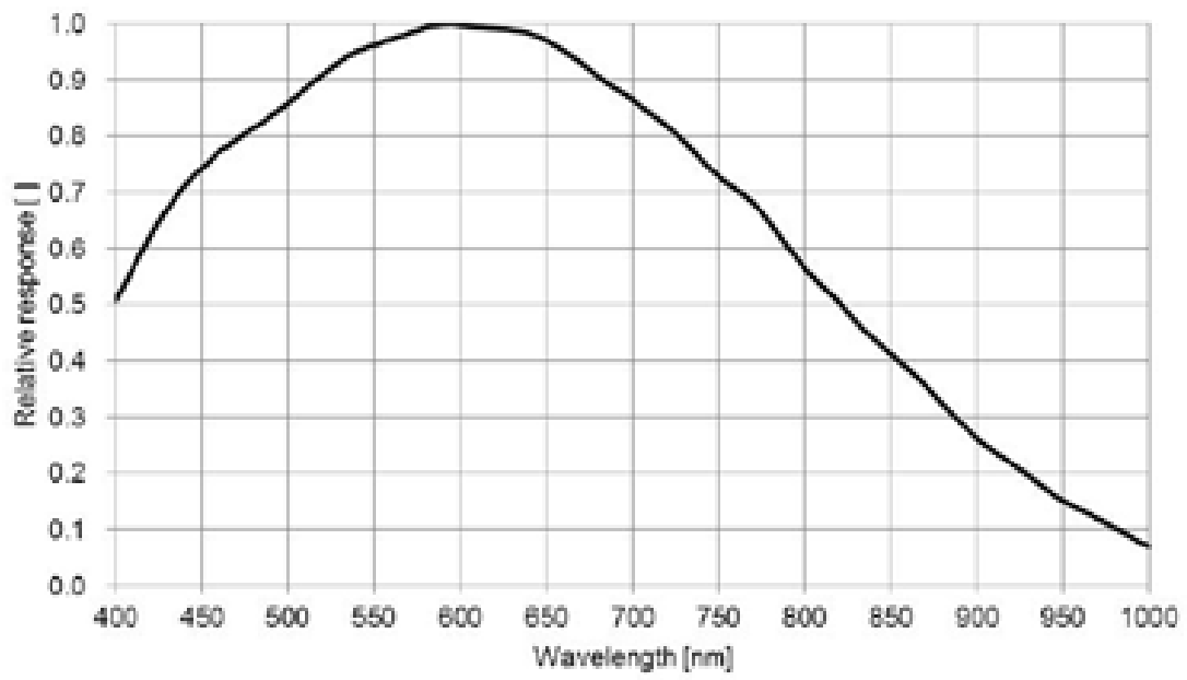
MER2-301-125U3M 光谱曲线
