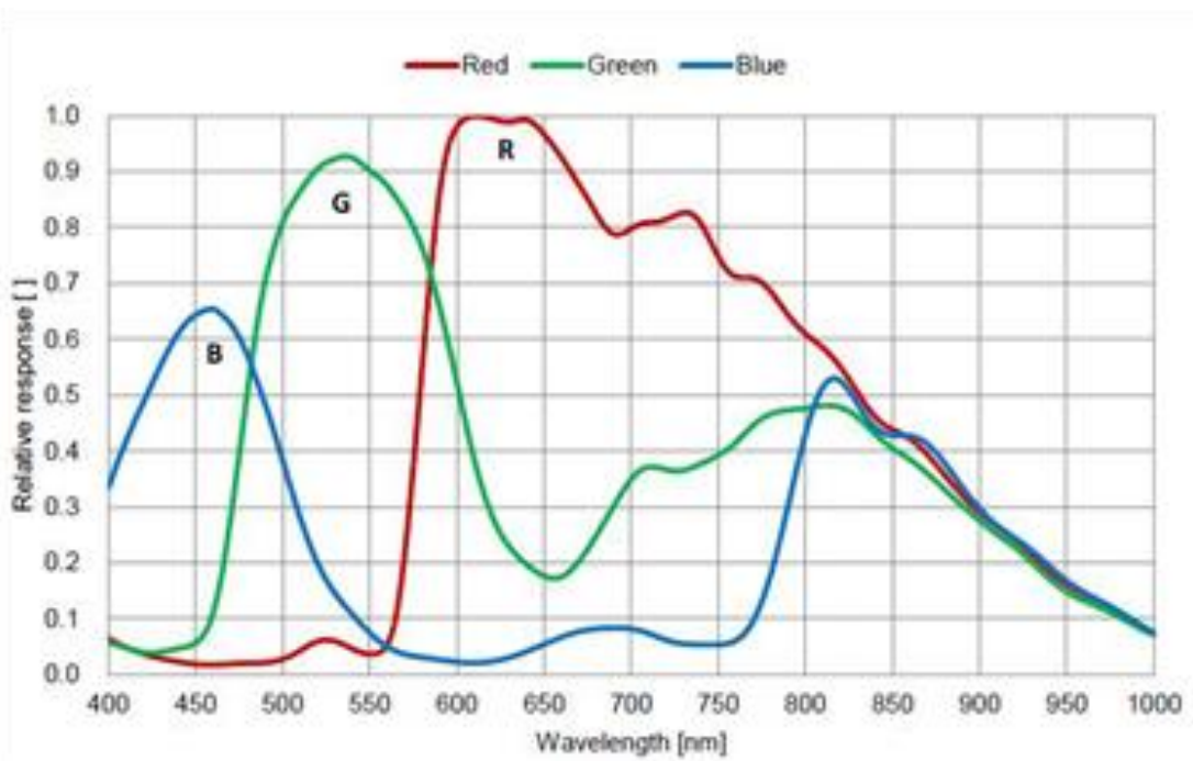
MER2-301-125U3C 光谱曲线
